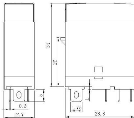
NNC69KTL-17 外形尺寸
